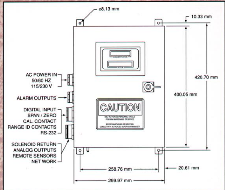
3010TBC & 3010PBC
