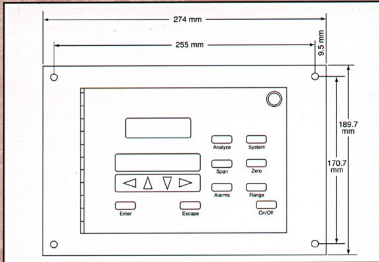
3010TAC & 3010PAC
